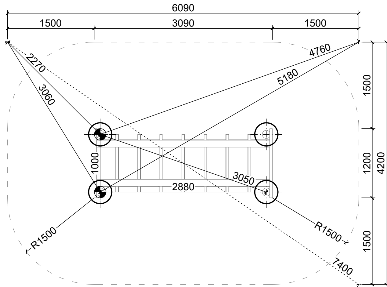
Osově symetrický prvek
