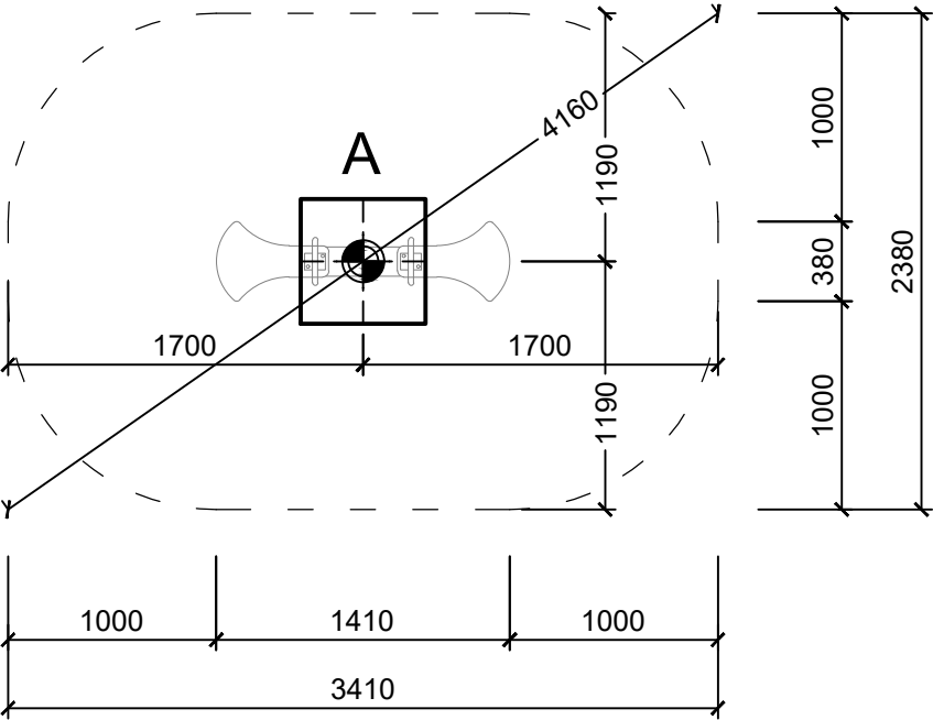
PŮDORYS HERNÍHO PRVKU
